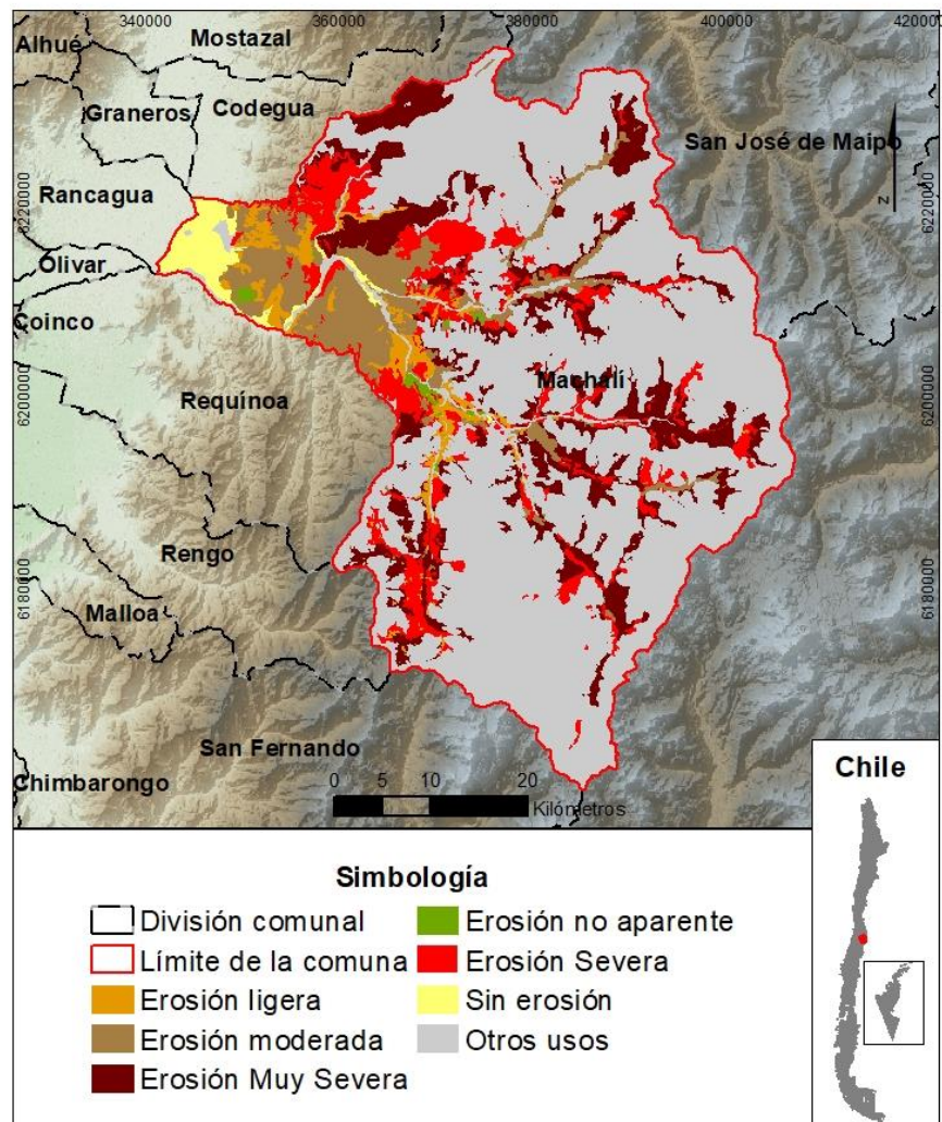
Distribución espacial de la Erosión Actual
