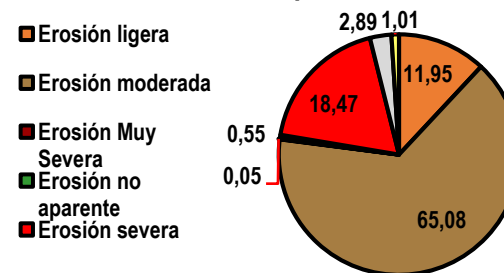
Distribución porcentual de Erosión
