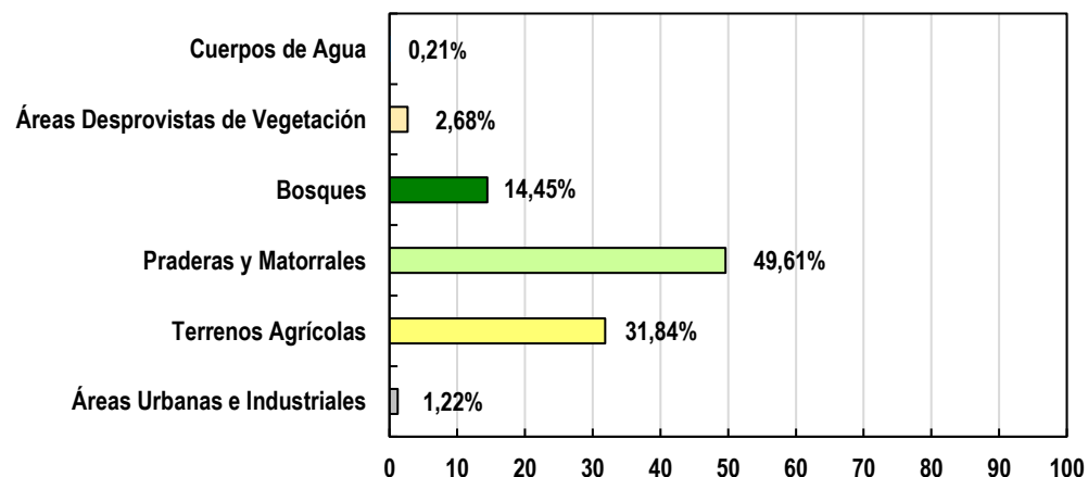
Distribución porcentual de los Usos de la Tierra
